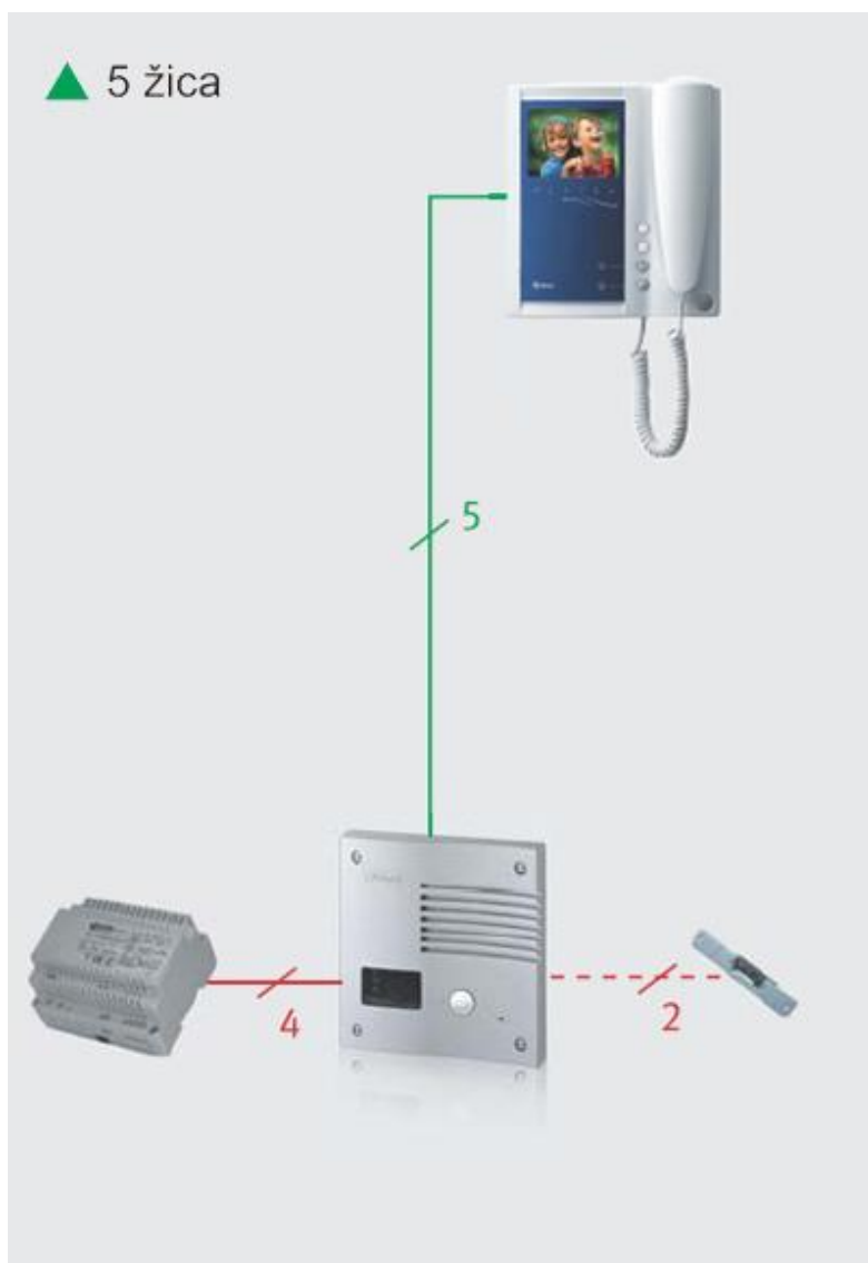
Povezivanje video interfonskog sistema sa 5 žica
