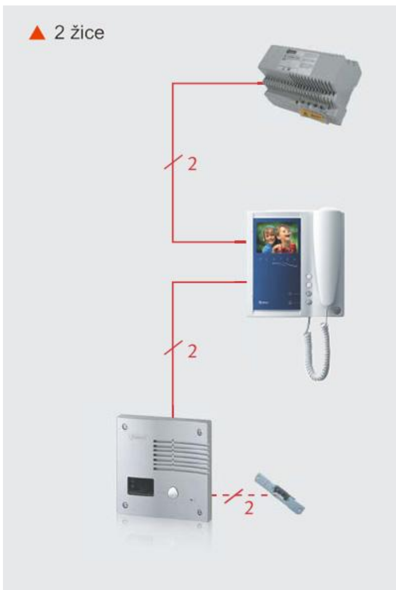
Povezivanje video interfonskog sistema sa 2 žice
